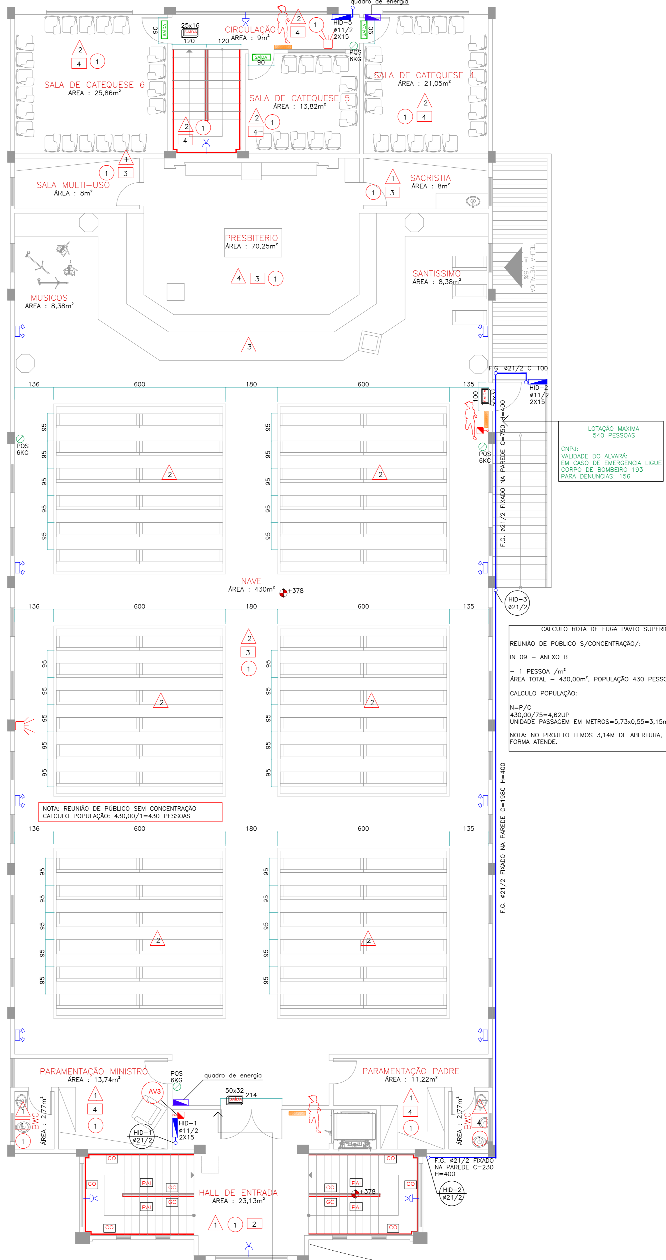
PLANTA BAIXA PREVENTIVO - SUPERIOR 1/75
