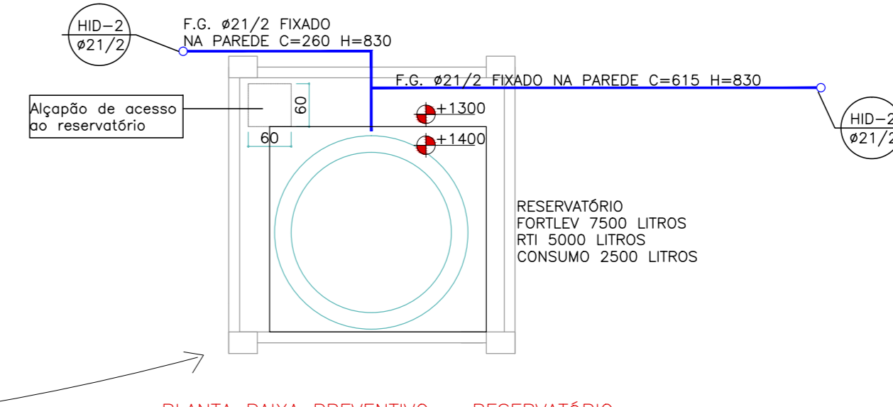
PLANTA BAIXA PREVENTIVO - RESERVATÓRIO 1/75
